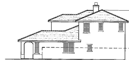
Right Elevation
